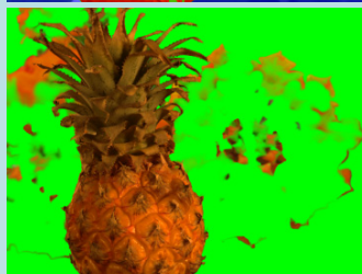
[Juan & Keriven '06] (13.4;13.6)
