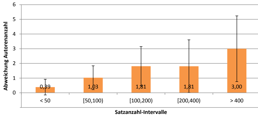
Abbildung 5.6: Abweichung der ermittelten Clusteranzahl \pm \sigma bezüglich der Textlänge (gruppiert nach Satzanzahl-Intervallen).
