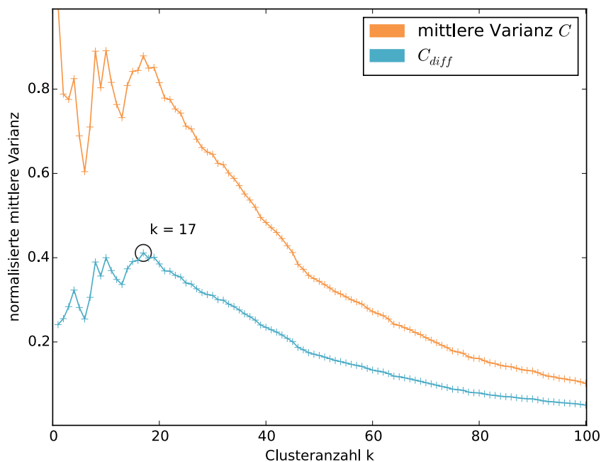
Abbildung 5.9: Knee Point Detection mit globalem Maximum bei k = 17 und zwei ähnlich ausgeprägten Punkten an den Stellen k = 8 und k = 10 . Der Testdatensatz wurde von 8 Autoren verfasst, das Qualitätsmaß für die ermittelte Clusteranzahl (17) beträgt 0,21.
