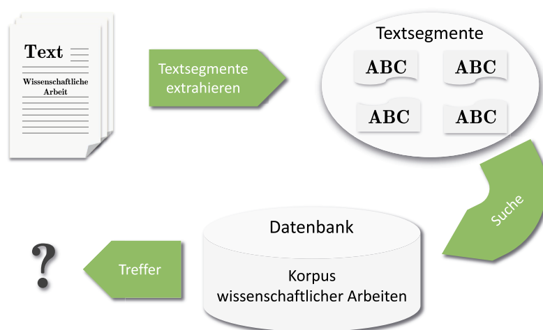
Abbildung 2.1: Ablauf korpusbasierter Plagiatserkennung.
