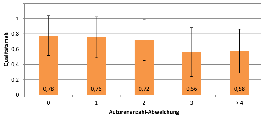
Abbildung 5.10: Qualitätsmaß der ermittelten Clusteranzahl \pm \sigma . Ab einer Abweichung von 3 ist eine deutliche Senkung erkennbar.
