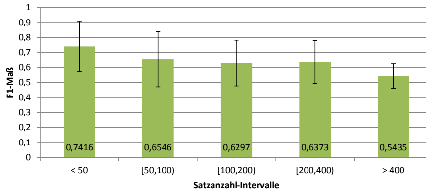
Abbildung 5.7: F1-Maß \pm \sigma gruppiert nach Satzanzahl-Intervallen.
