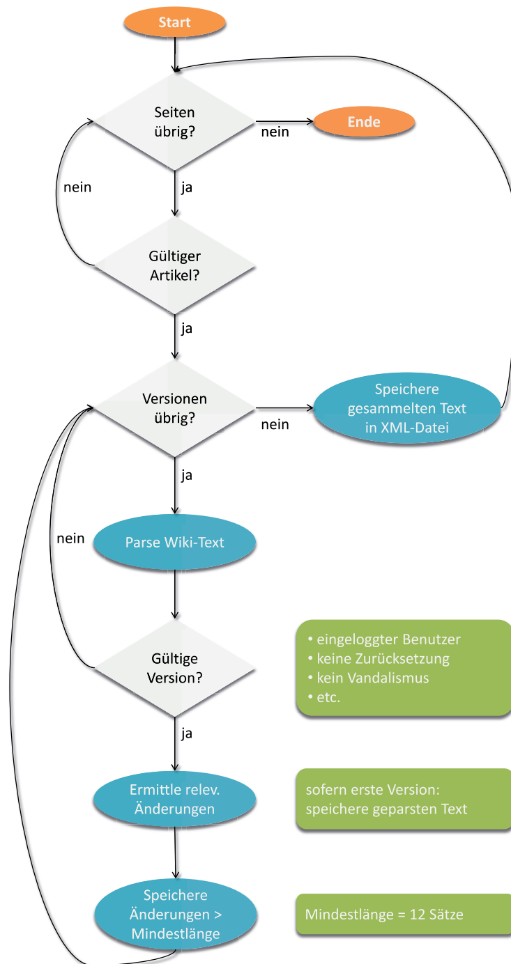
Abbildung 4.2: Verarbeitungsablauf einer Wikipedia-Datenbank-Dumpdatei.
