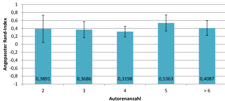
Abbildung 5.5: Angepasster Rand-Index \pm \sigma gruppiert nach Autorenanzahl.
