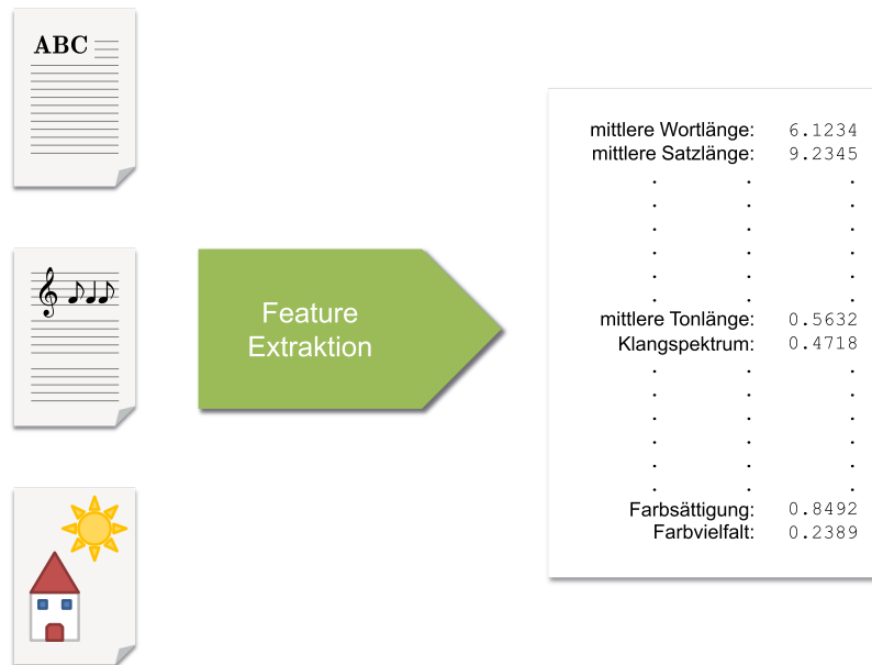
Abbildung 2.2: Stilometrische Features aus Dokumenten extrahieren.
