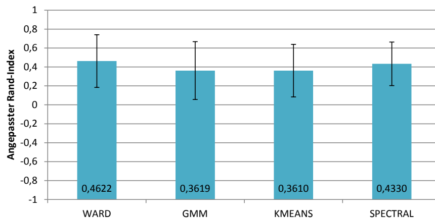
Abbildung 5.2: Clusterperformance mit vorgegebener Autorenanzahl: mittlerer angepasster Rand-Index \pm \sigma . Testdaten mit nur einem Autor wurden ignoriert.
