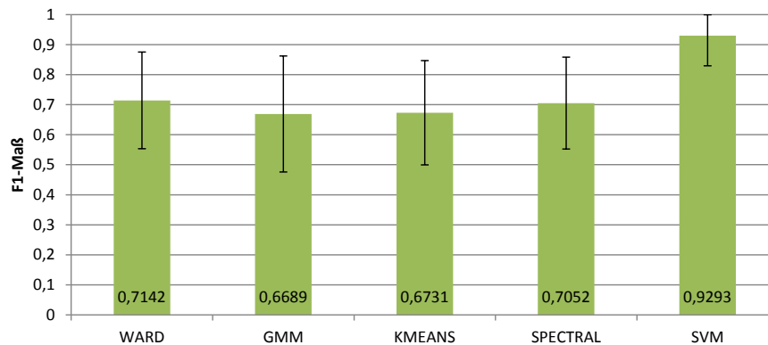
Abbildung 5.1: Clusterperformance mit vorgegebener Autorenanzahl und Performance einer SVM im Vergleich: mittleres F1-Maß \pm \sigma . Testdaten mit nur einem Autor wurden ignoriert.
