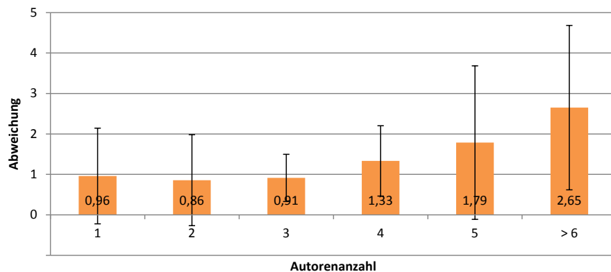
Abbildung 5.3: Abweichung der ermittelten Clusteranzahl \pm \sigma gruppiert nach Autorenanzahl.
