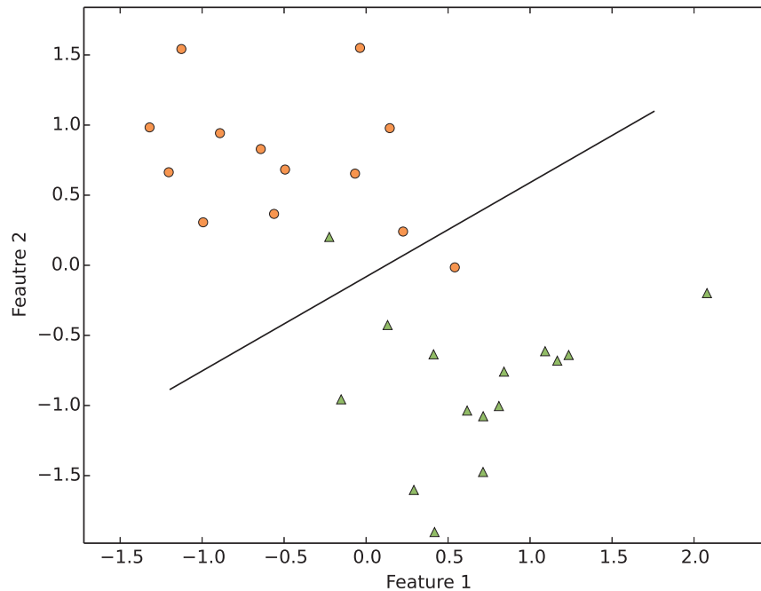
Abbildung 2.4: Datenpunkte zwei verschiedener Klassen in einem zwei-dimensionalen Vektorraum. Die schwarze Linie stellt eine mögliche Entscheidungsgrenze dar (jeweils ein Datenpunkt würde der falschen Klasse zugeordnet werden).
