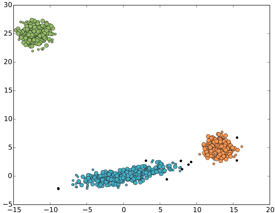
Abbildung 3.5: DBSCAN ( \epsilon = 1.0 , minPts = 10 ): drei Cluster gefunden. Randpunkte werden im Vergleich zu den Kernpunkten kleiner dargestellt. Punkte in schwarz sind Rauschpunkte.
