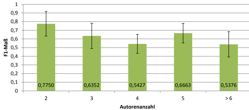
Abbildung 5.4: F1-Maß \pm \sigma gruppiert nach Autorenanzahl.
