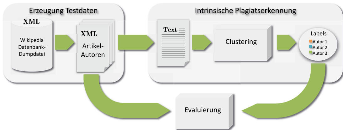
Abbildung 4.1: Gesamter Ablauf: Erstellung Testdaten, intrinsische Plagiatserkennung und Evaluierung.
