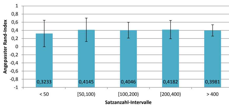
Abbildung 5.8: Angepasster Rand-Index \pm \sigma gruppiert nach Satzanzahl-Intervallen).
