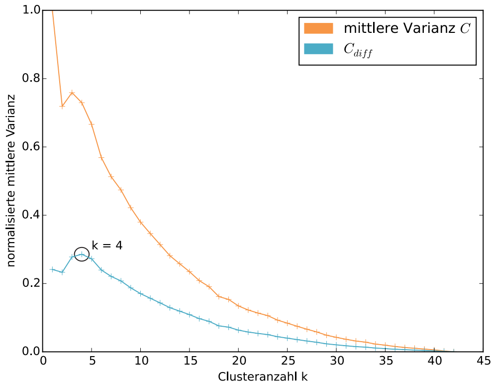
Abbildung 4.4: Ermittlung der Clusteranzahl k über den Vergleich mit der fallenden Varianz. Die C_{diff} -Kurve wird in blau dargestellt und befindet sich unter der C -Kurve. Die tatsächliche Klassenanzahl dieser Testdaten beträgt 5 und das Qualitätsmaß 0,9091.
