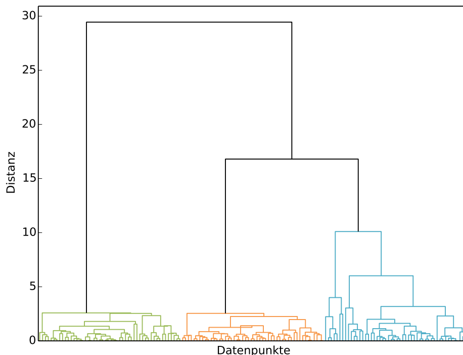
Abbildung 3.3: Dendrogramm eines hierarchischen Clusterings mit Average Linkage: die drei eingefärbten Unterbäume stellen eine mögliche Clusteraufteilung dar.
