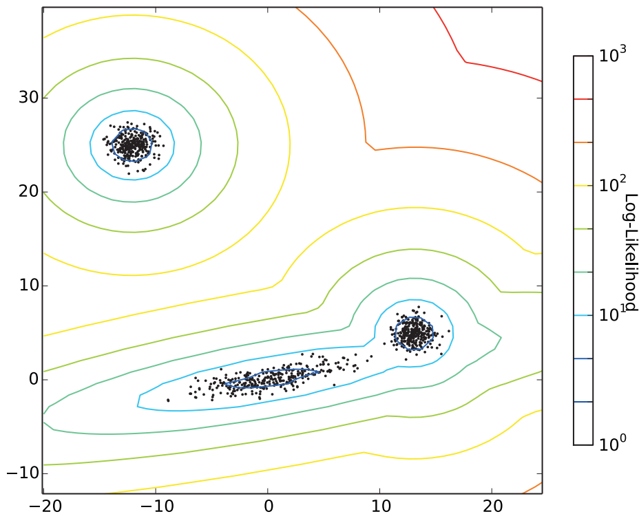
Abbildung 3.4: Dichteverteilungskurven eines GMM mit drei Komponenten.
