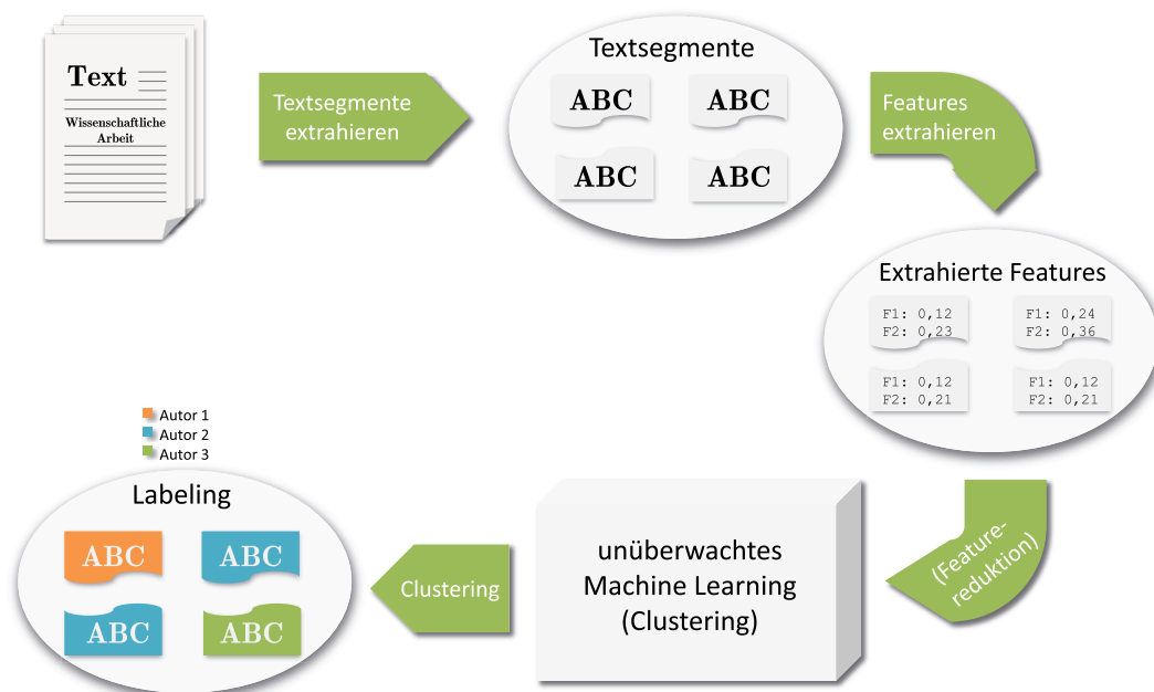
Abbildung 2.3: Möglicher Ablauf einer stilometrischen Plagiatserkennung.
